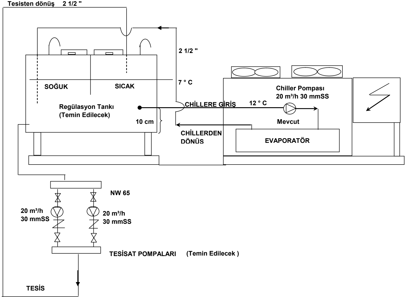
PROSES SOĞUTMADA CHILLER GRUBUNUN REGÜLASYON TANKINA ÇALIŞMASI PRENSİP ŞEMASI
