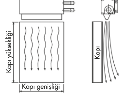
Kapı üstü Montajı Maksimum 2 - 3 m Şekil - 1 Endüstriyel tip ve Ticari tipler için
