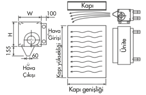
Kapı yanı Montajı Maksimum 4 - 6 m Şekil - 2 Endüstriyel tipler için
